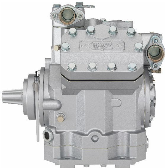
Afbeelding 2: De 4-cilinder ROADSTAR 4GFC(Y) is net zo krachtig als een 6-cilinder – maar veel compacter
